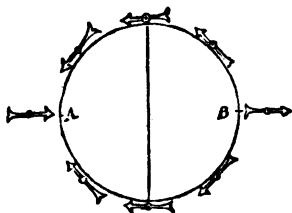
Fig. 1. GILBERT'S TERRELLA.
